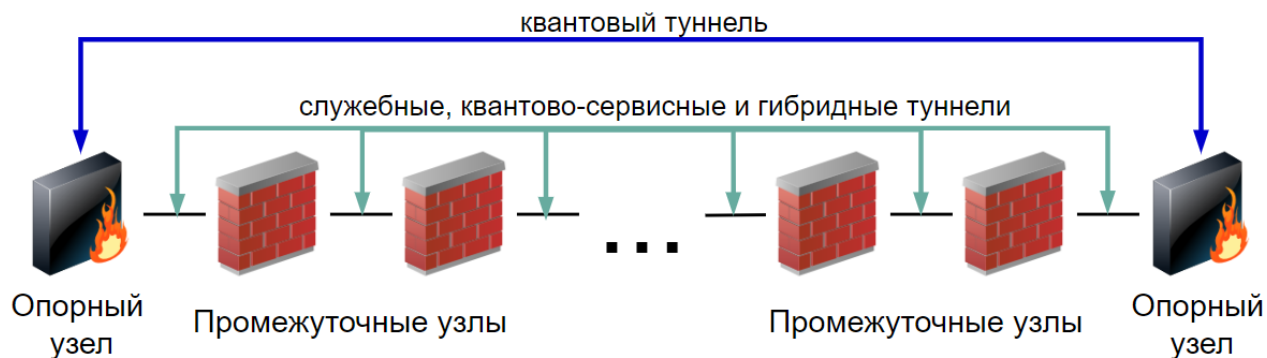
Рисунок 273 - Общая схема линейной квантовой сети
